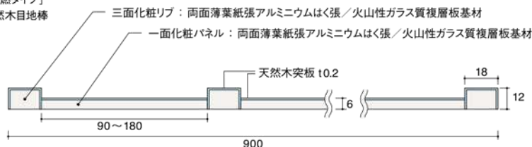
断面図
