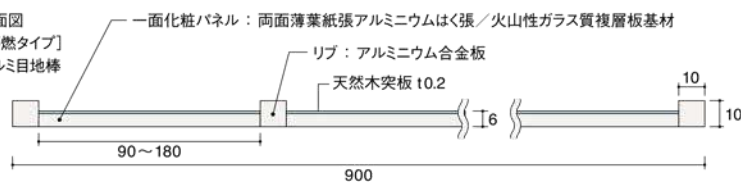
断面図
